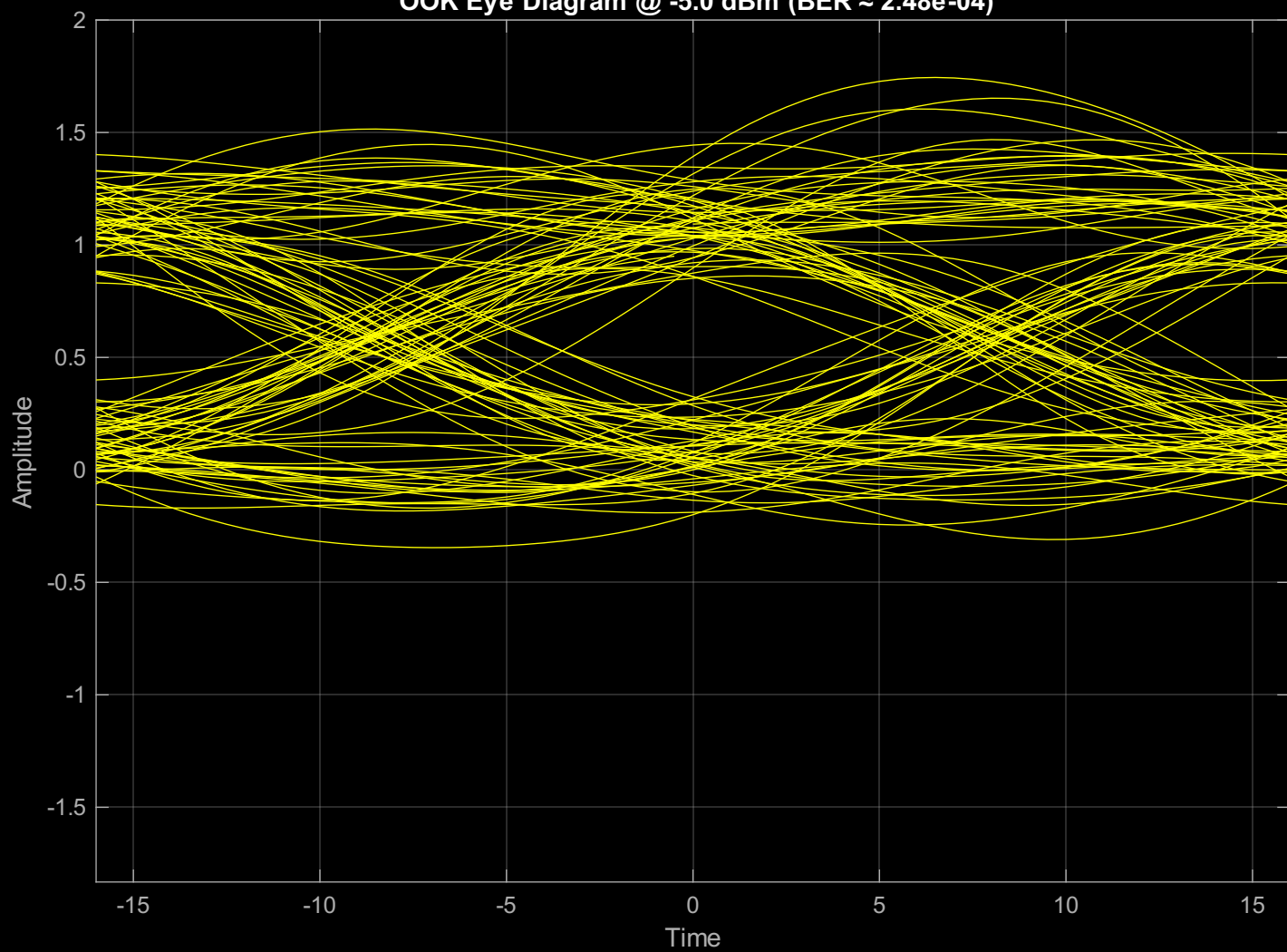
OOK Eye Diagram @ -5.0 dBm (BER \approx 2.48\text{e-}04 )
